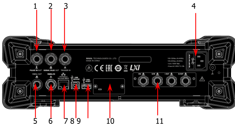
Рисунок 2. Задняя панель
